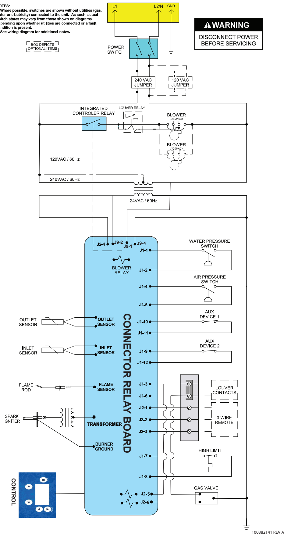
Figure 10-3_Diagramme en escalier
