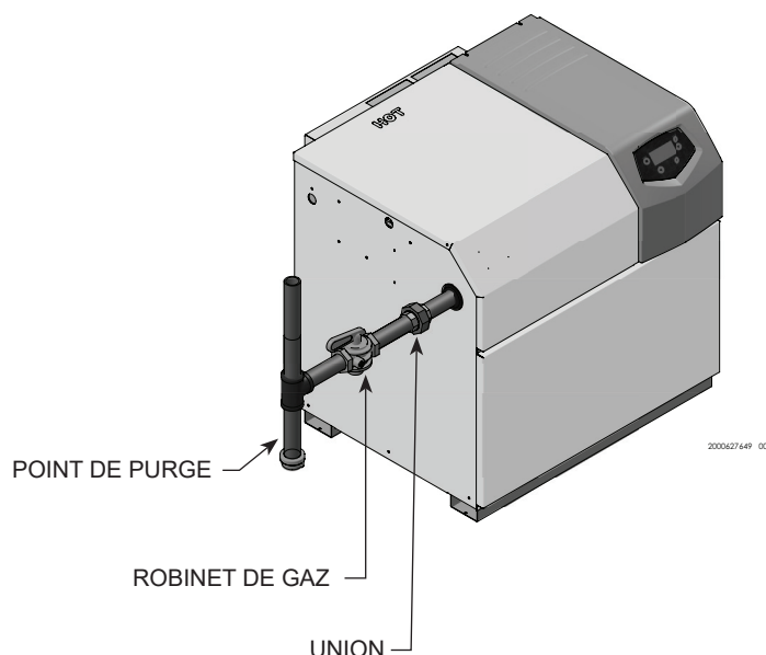
Figure 6-1 Raccordement de la conduite de gaz à l'appareil avec piège à sédiment et vanne principale d'arrêt manuel du gaz
