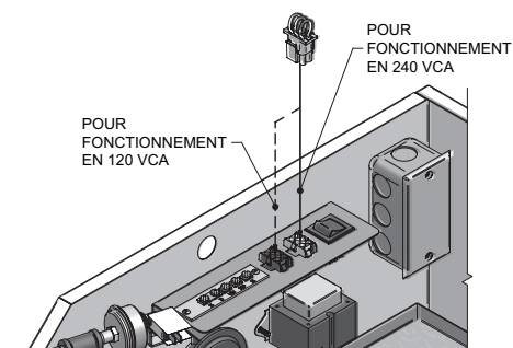
Figure 8-1_Cavalier de tension - 240 VCA à 120 VCA
