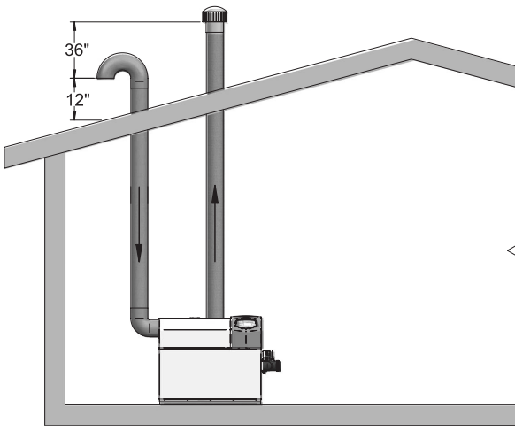
Figure 2-3 Ventilation DirectAire verticale avec entrée d'air verticale - Voir page 20 pour davantage de détails
