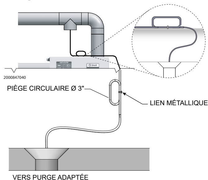
Figure 5-7 _ Installation du té de purge
