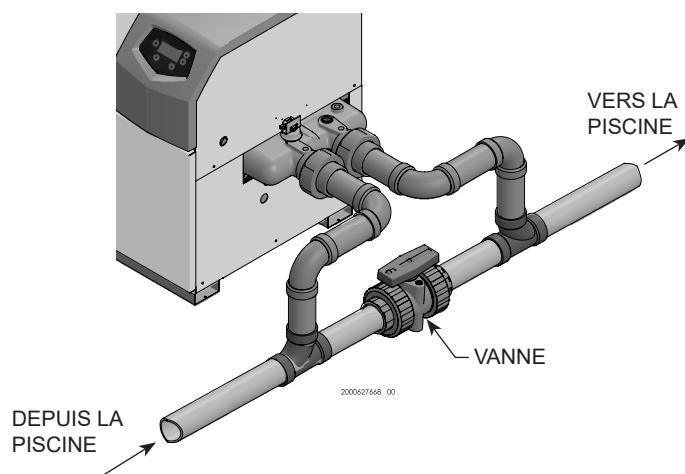
Figure 7-3_ Tuyauterie de dérivation auxiliaire
