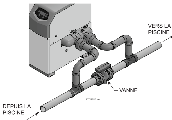
Figure 11-2_ Tuyauterie de dérivation auxiliaire
