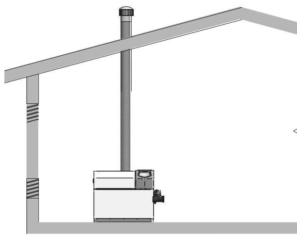
Figure 1-2 Air de combustion direct de l'extérieur
