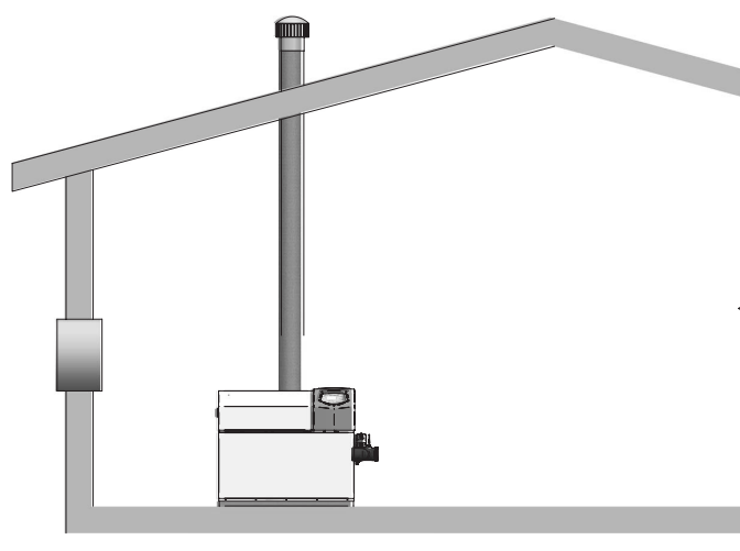
Figure 1-5 _Air de combustion de l'extérieur - Ouverture unique
