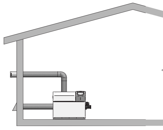
Figure 5-5_Installation d'une ventilation E-Rite latérale
