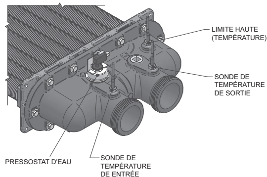
Figure 8-4_Collecteur avant avec limites
