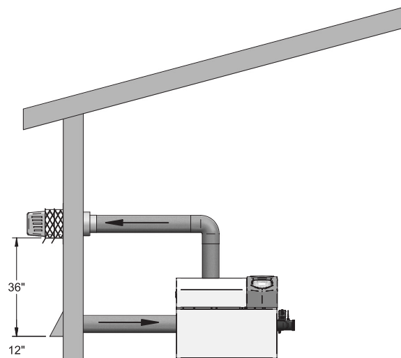
Figure 5-3_Illustration de l'installation électrique DirectAire horizontale
