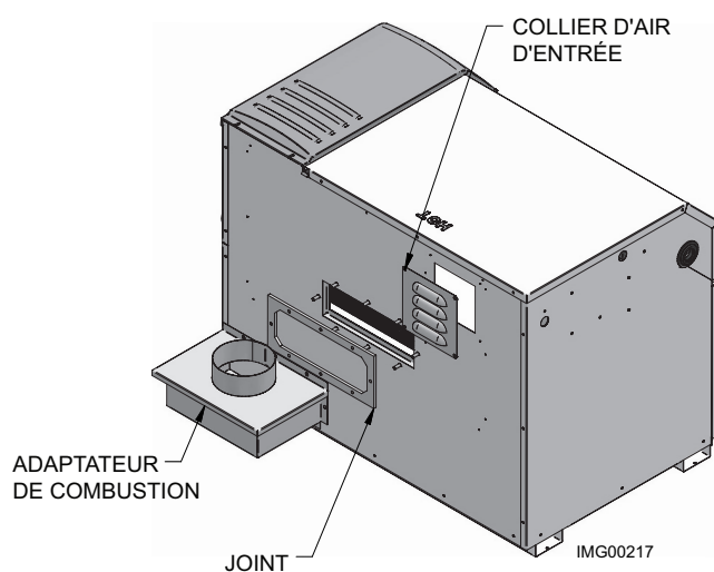
Figure 2-12_Installation d'un adaptateur de fumées et d'un couvercle d'entrée d'air
