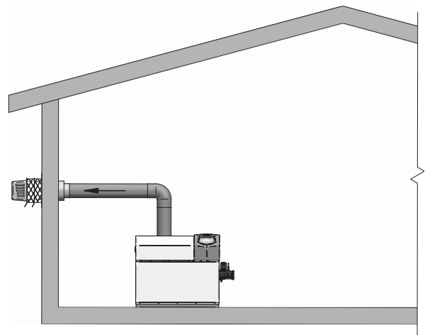
Figure 2-4 Ventilation électrique latérale - voir page 24 pour davantage de détails
