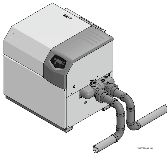
Figure 7-2 Tuyauterie classique pour raccordement d'eau
