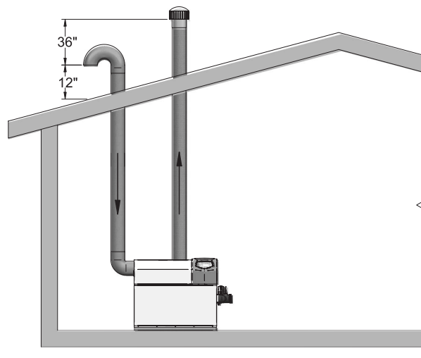
Figure 4-7 Installation DirectAir verticale avec air de combustion par le toit
